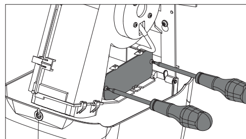
Platinenabdeckung demontieren
