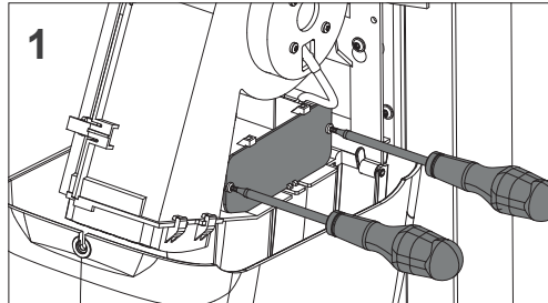
Platinenabdeckung demontieren
