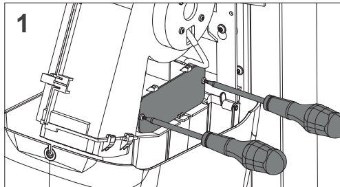
Platinenabdeckung einsetzen und festschrauben.
