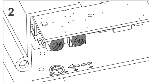
Zeiteinstellung Potentiometer Im Uhrzeigersinn drehen, maximum (5 Min.) Gegen Uhrzeigersinn drehen, minimum (30 Sek.) Annäherungseinstellung Potentiometer Im Uhrzeigersinn drehen, maximum (15 cm) Gegen Uhrzeigersinn drehen, minimum (10 cm)
